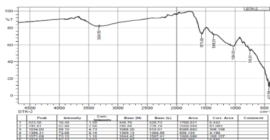
Gambar 3. FTIR Biochar tempurung kelapa
