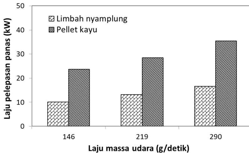
Gambar 8. Laju pelepasan panas pembakaran limbah nyamplung dan pelet kayu pada burner.
