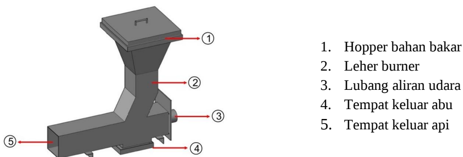
Gambar 3. Hasil rancangan burner biomassa.
