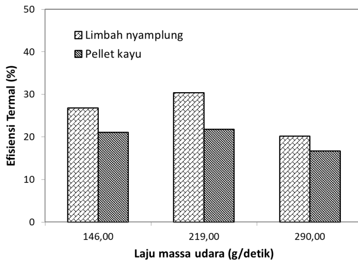
Gambar 9. Efisiensi termal pembakaran burner biomassa menggunakan limbah nyamplung dan pelet kayu.
