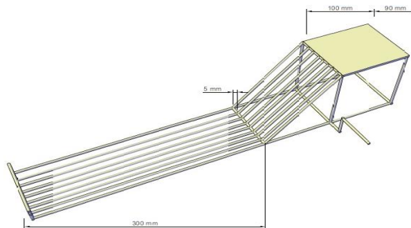
Gambar 5. Desain rangka pembuangan abu.
