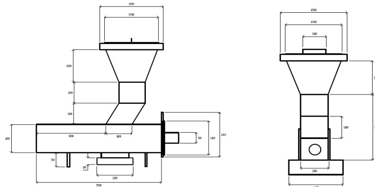
Gambar 4. Gambar tampak depan dan tampak samping desain 2D burner biomassa.
